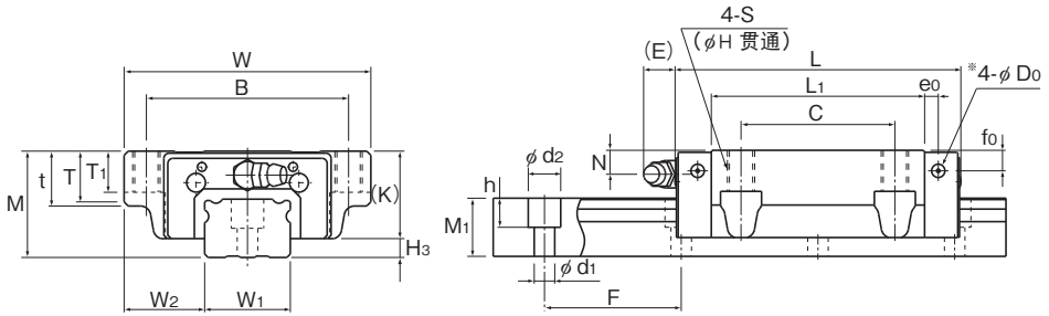
SNR-C型
