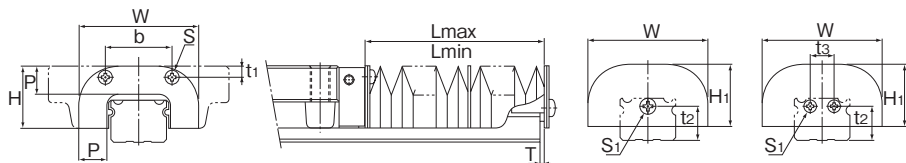
SNR25~45型
