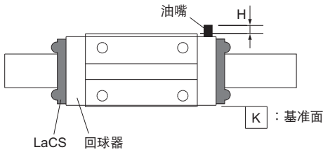
SHS、SSR、SVR/SVS、SNR/SNS、SRG和NR/NRS型 油嘴安装部位
