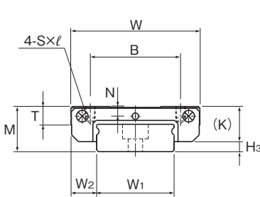
SRS7WM/9、12WM/WN型
