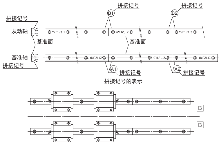
图4 拼接使用
