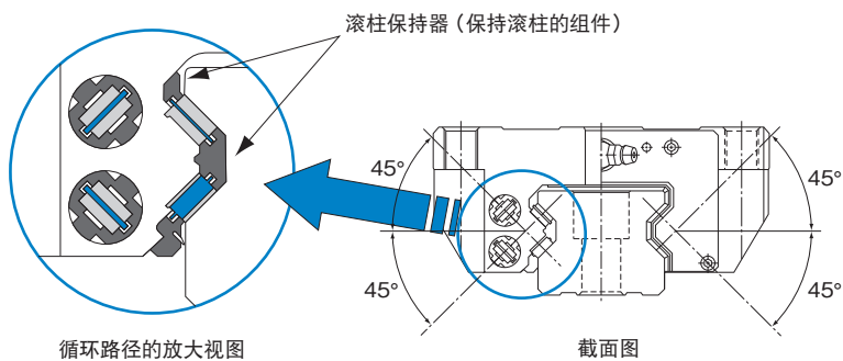
图1 保持器型滚柱滚动导轨SRG型的结构图
