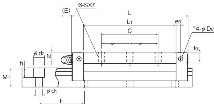
SNS-LR型
