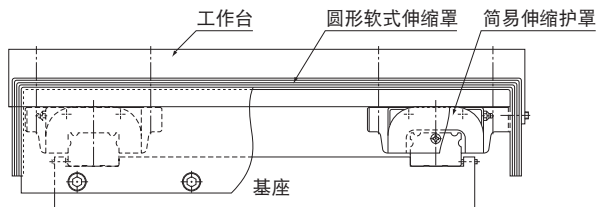
图1 装配简易伸缩护罩例
