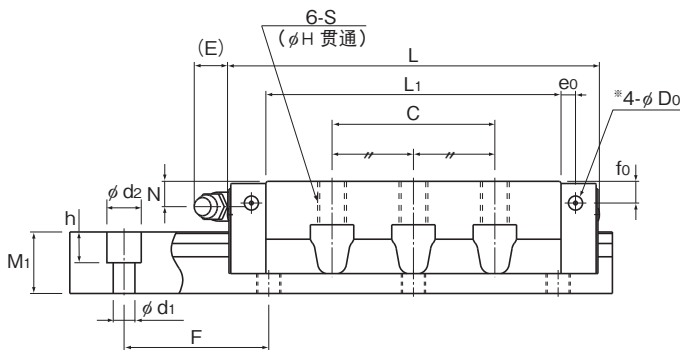
SNR-LC型
