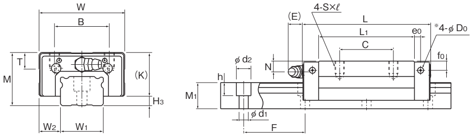
SNS-R型
