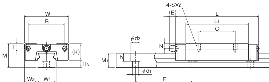
RSR15、20M1V/M1N型
