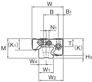
GSR15T/V型
