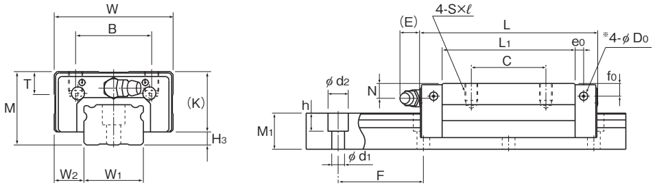
SNR-R型
