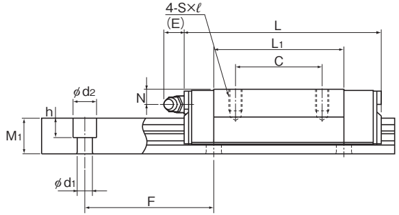
GSR15~35T型
