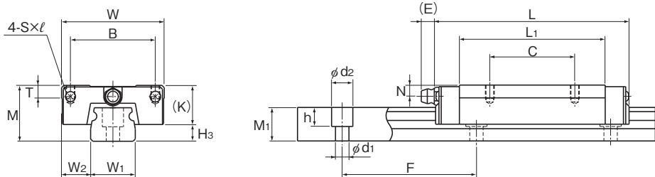
RSR15、20VM/N型
