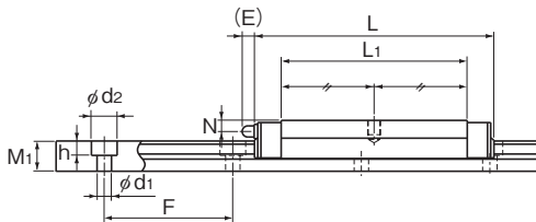
RSR5WTM/WTN型
