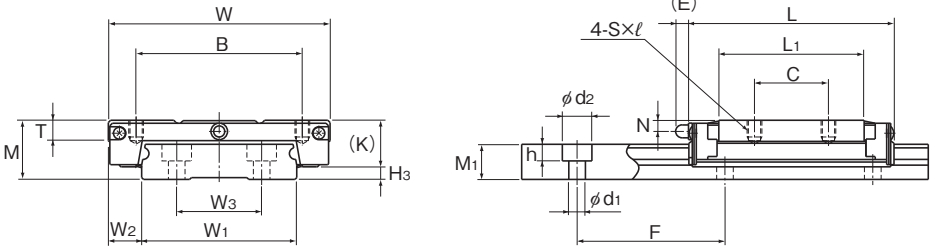
RSR15WZM型
