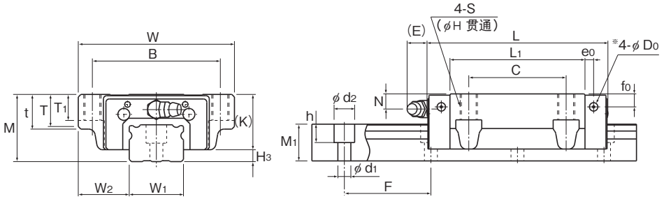
SNS-C型
