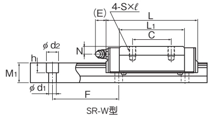
SR-W型
