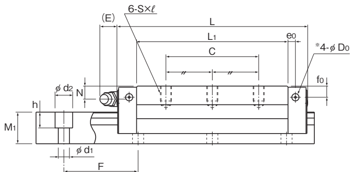
SNR-LR型
