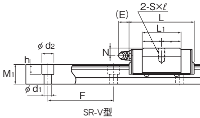
SR-V型
