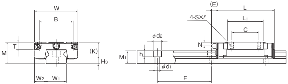
RSR15ZM型
