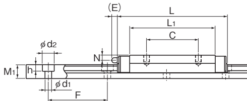
RSR15WV/WVM/WN型
